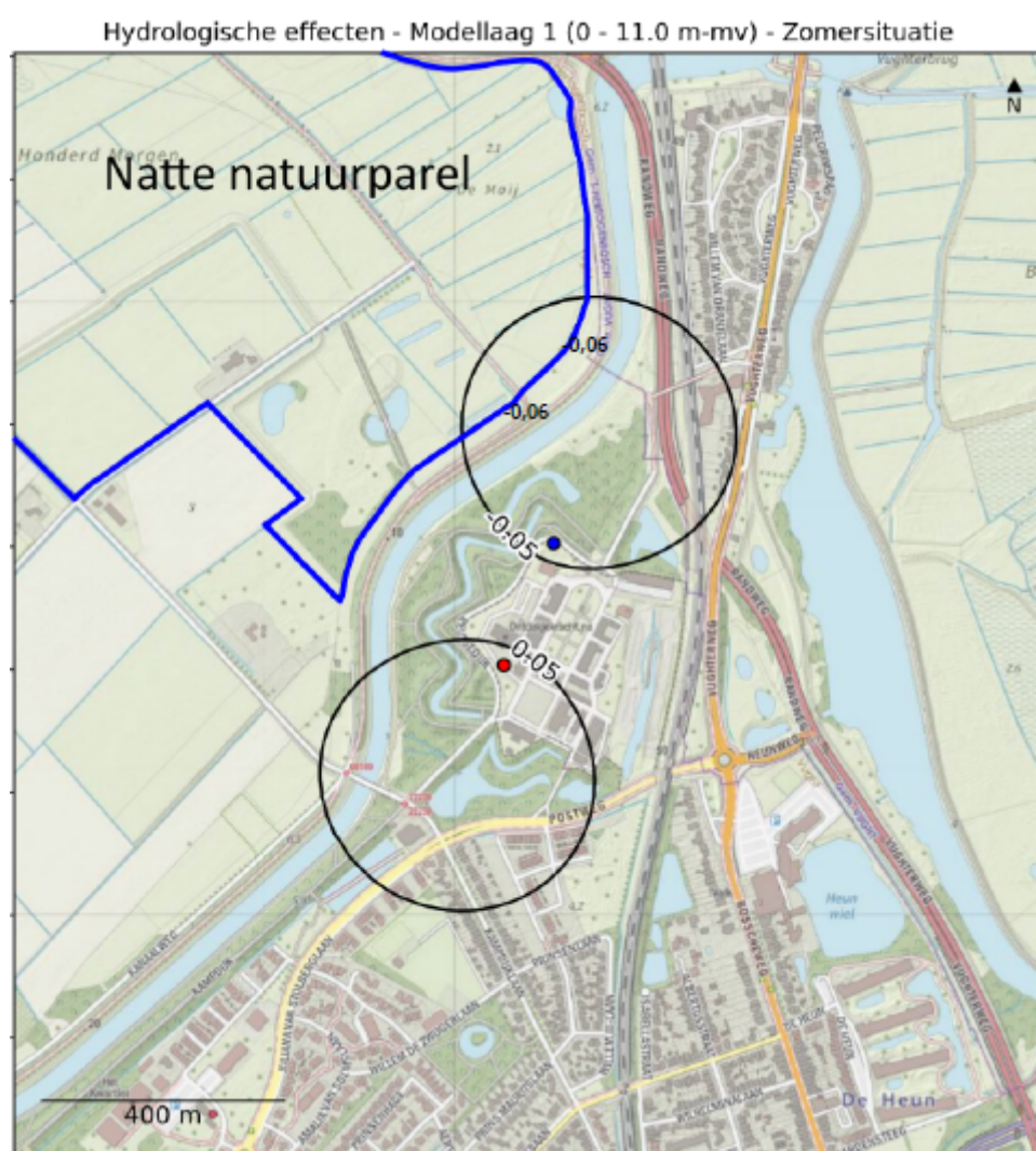
Figuur 2. Hydrologisch invloedsgebied freatisch pakket en locatie natte natuurparel.
