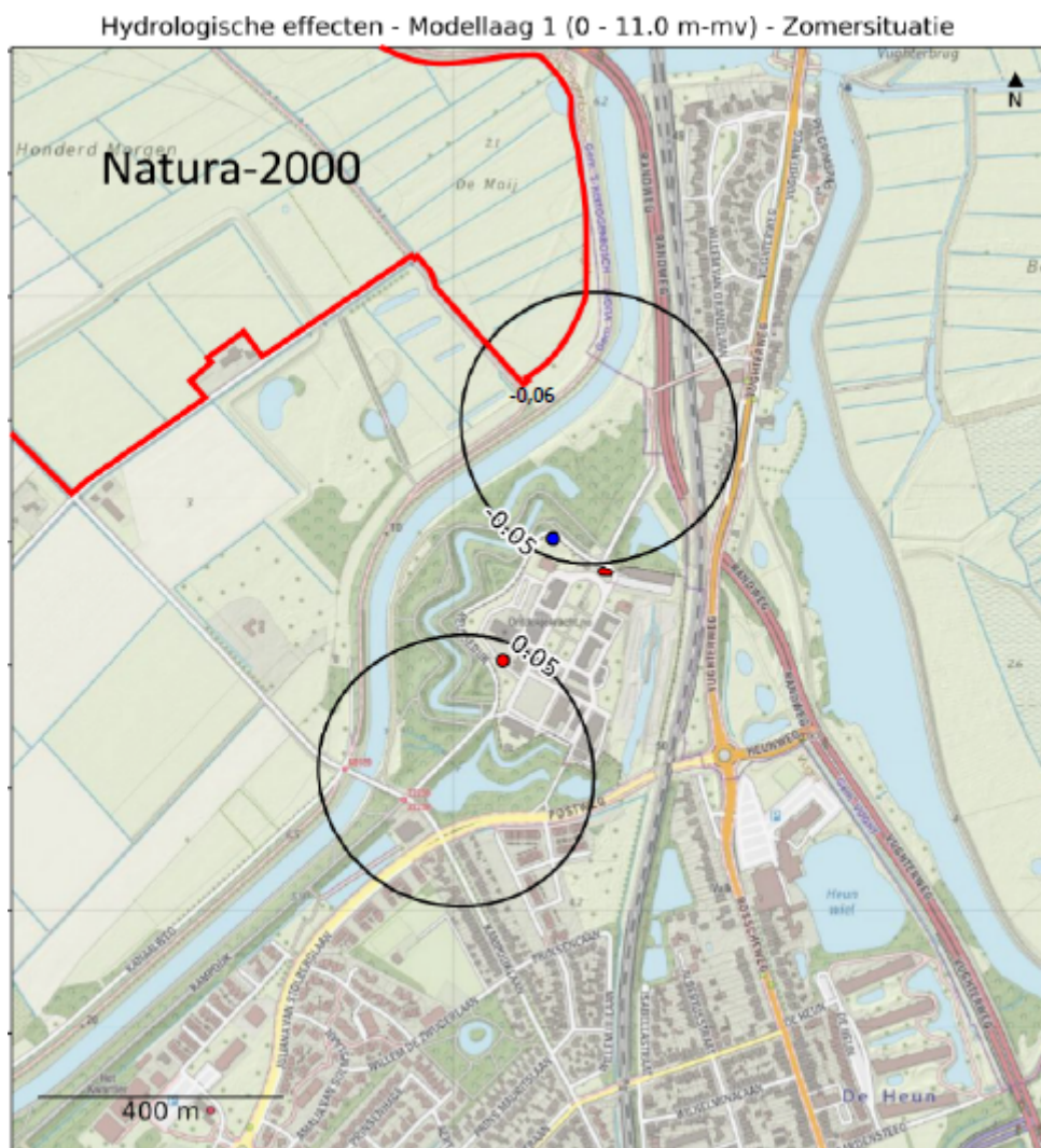
Figuur 1. Hydrologisch invloedsgebied freatisch pakket en locatie Natura 2000 gebied.
