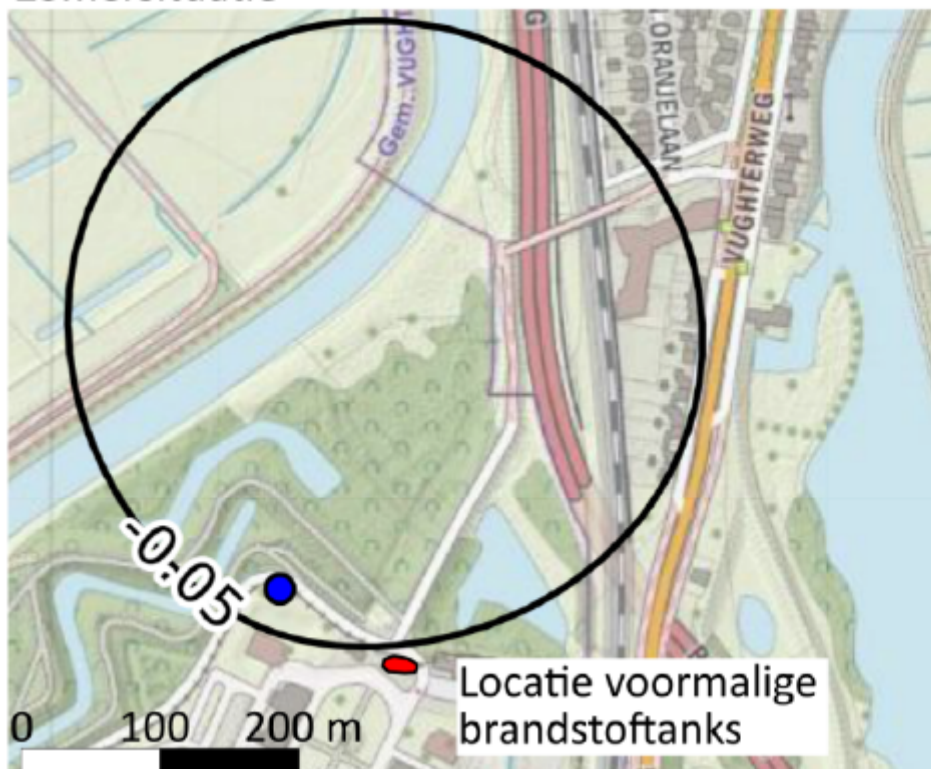
Figuur 3. Hydrologisch invloedsgebied freatisch pakket en locatie voormalige brandstoftanks.
