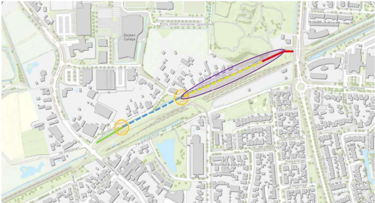
Figuur 1. Locatie Geerbosch (nabij Gasthuisstraat 47), Veghel. De locaties waar duikers vervangen en verlengd worden zijn aangegeven met de oranje cirkels. De locatie waar de watergang gedempt en verplaatst zal worden, wordt aangegeven met de paarse cirkel. De groene lijn geeft aan waar eDNA van de grote modderkruiper is aangetroffen en de rode lijn geeft aan waar dit niet het geval is. Bij de blauwe stippellijn komt de soort vermoedelijk voor en bij de gele stippellijn wordt de soort niet verwacht.
