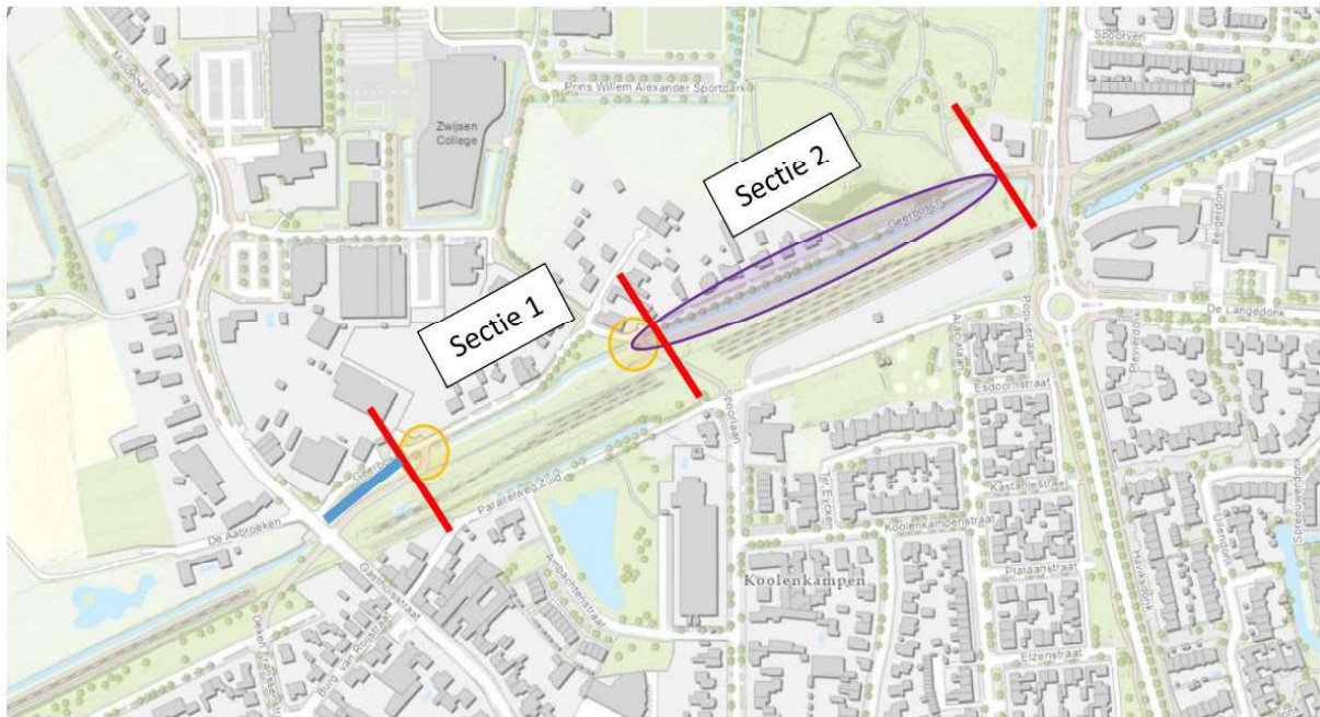
Figuur 2. Locatie van de maatregelen. De oranje cirkels geven de te vervangen duikers weer, de paarse cirkel de te vergraven watergang. De rode lijnen symboliseren waar de watergang opgebroken zal worden. De blauwe lijn geeft geschikt habitat weer om eventuele afgevangen dieren in over te zetten.
