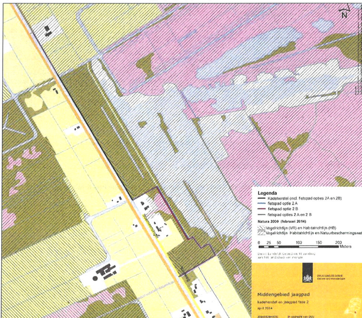
Figuur 1. Locaties van de te herstellen kade en het aan te leggen fietspad (optie 2b).
