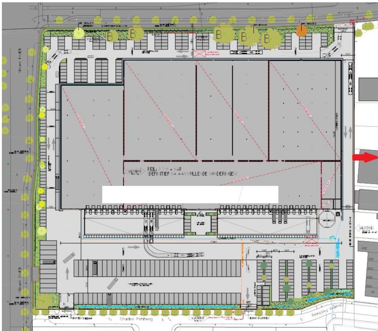
Figuur 2-4. Concept weergave terreintekeningen toekomstige Sligro Bezorgservice en Distributiecentra inclusief bomenplan op de planlocatie aan de Kapittelweg 10 te Breda (Architect Omni, Situatie Wabo 16-07-2018, schaal: 1:500). Noorden: rode pijl. Bron: Sligro.
