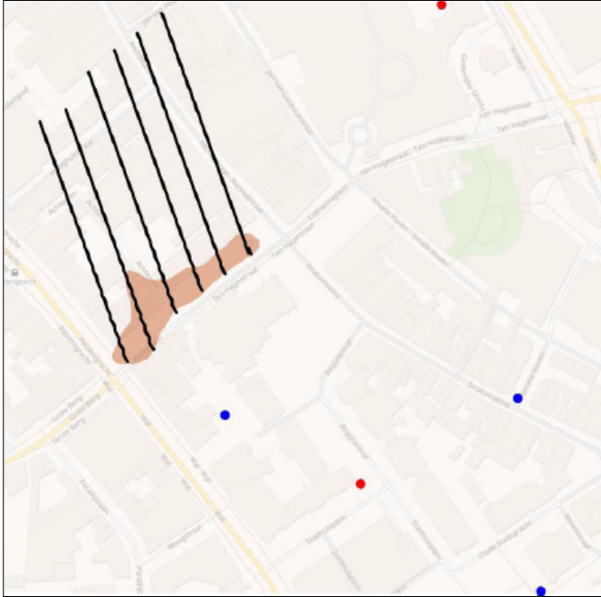
Figuur 2. Verplaatsing VOCl verontreiniging aan de Kerkstraat zonder invloed van het bodemenergiesysteem van Citywall
