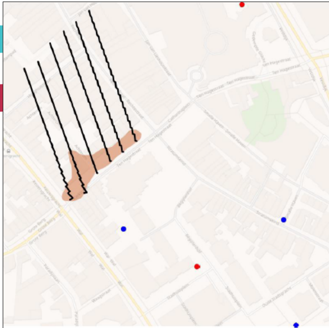
Figuur 3. Verplaatsing VOCl verontreiniging aan de Kerkstraat met invloed van het bodemenergiesysteem van Citywall
